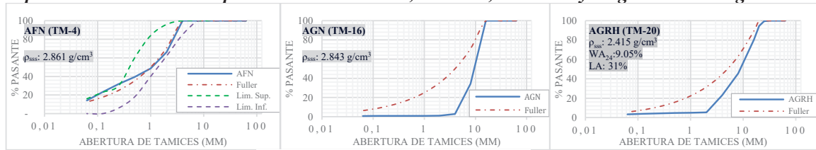
Figura 2. Resultados ensayos físicos AFN.
