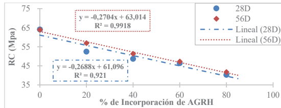
Figura 5. Resistencia a la compresión.
