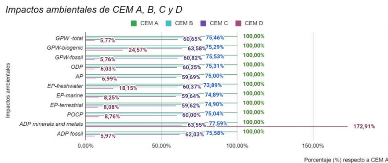
Figura 3. Comparación de los impactos ambientales entre los cementos analizados.
