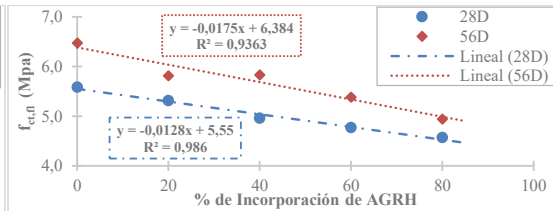
Figura 6. resistencia a la flexión.
