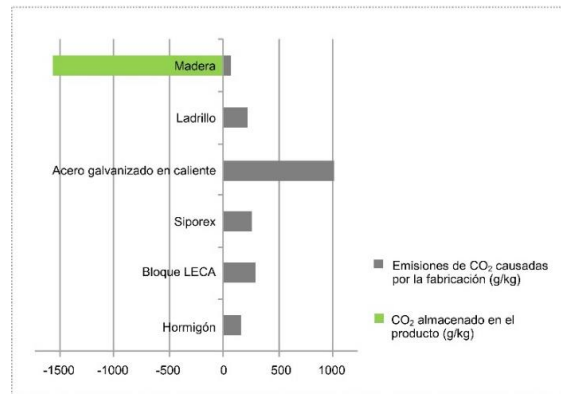
Figura 1. Emisiones de CO 2 causadas por la fabricación de diferentes materiales de la construcción y CO 2 almacenado en el material.
