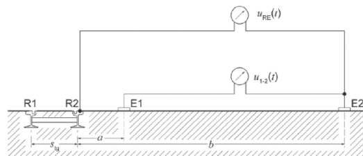
Figura 1. Esquema para la realización de las mediciones del ensayo de campo (UNE EN 50122-2:2023)
