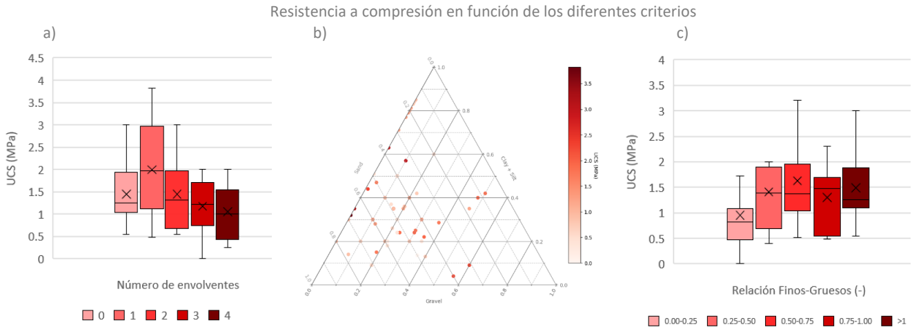
Figura 1. Resistencia a compresión en función de: a) el número de envolventes satisfechas, b) porcentaje de grava, arena y finos; c)
